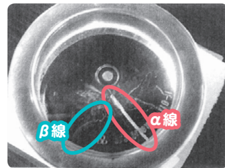
霧箱の写真
